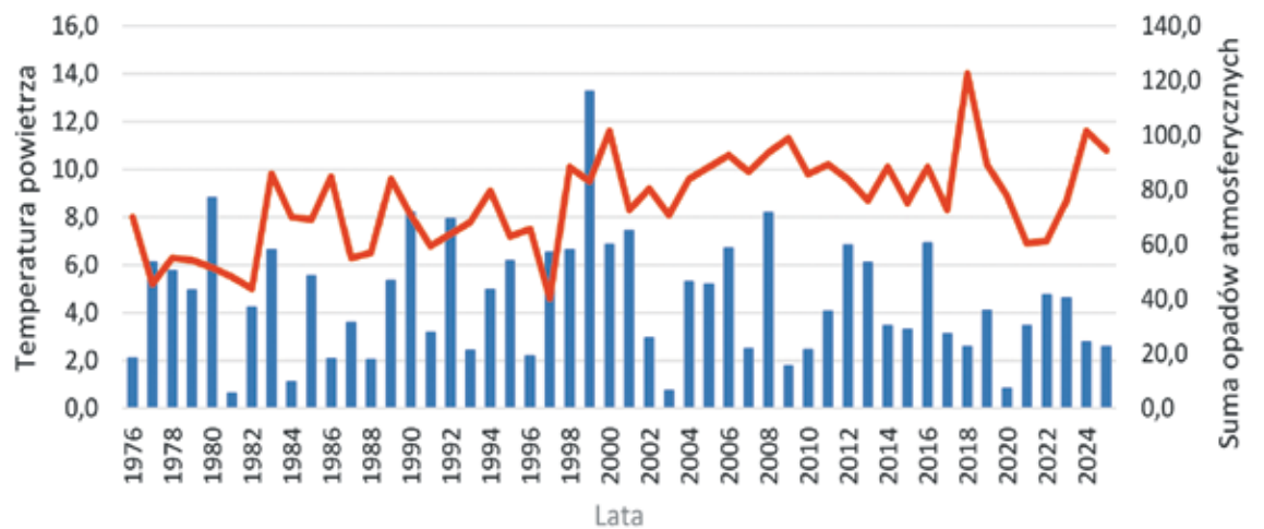
Temperatura powietrza i opady atmosferyczne w Zamościu, w kwietniu w latach 1976-2025
