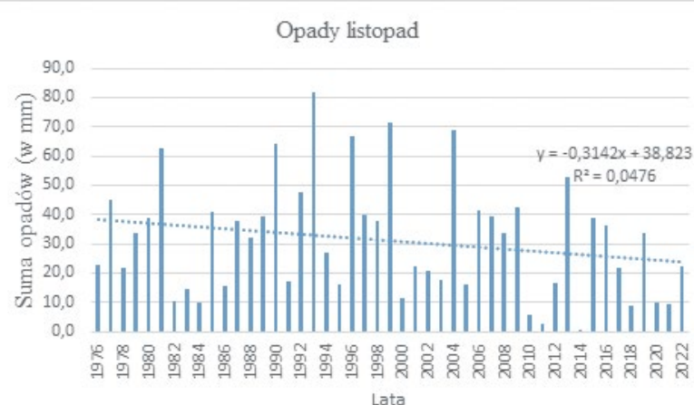
Suma opadów atmosferycznych w listopadzie (rys. dr hab. A. Samborski)
