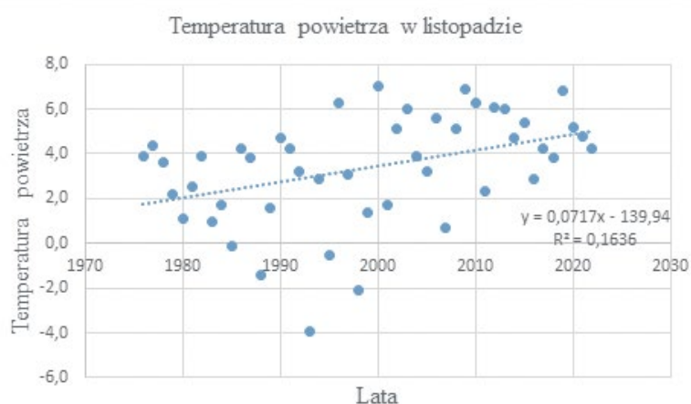
Temperatura powietrza w listopadzie (rys. dr hab. A. Samborski)
